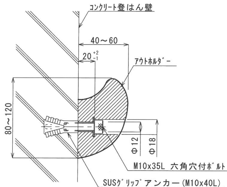
アウトホルダー取付詳細図 S=1/2
